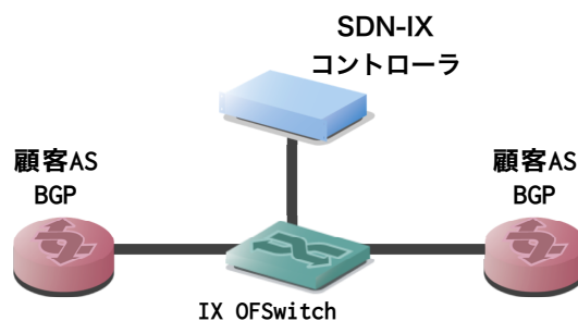
図 4 SDN-IX の構成
