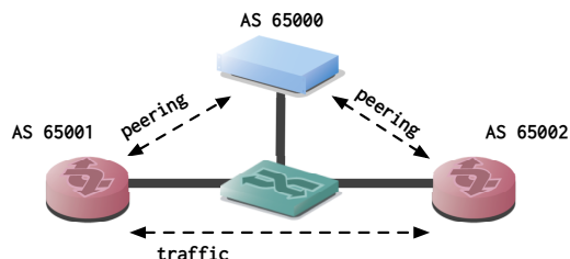
図 3 経路サーバ方式
