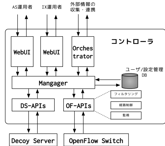
図 6 SDN-IX コントローラの構成
