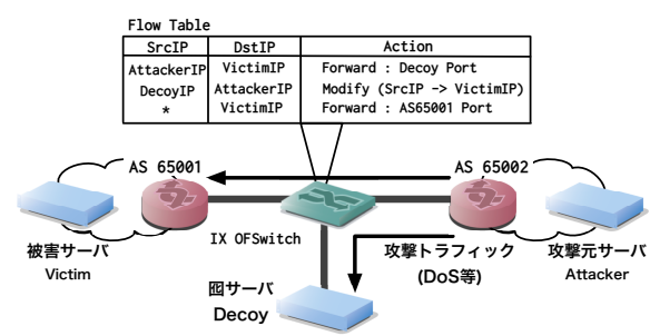
図 5 悪意のあるトラフィックの緩和
